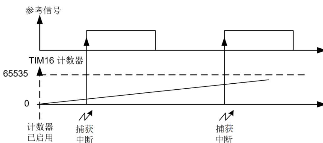
图 1.内部 RC 振荡器校准测量时序图
