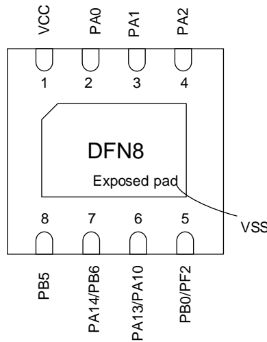
图 3-16 DFN8(1.5*1.5) Pinout1 PY32F030L1xD
