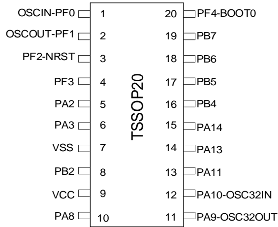
图 3-12 TSSOP20 Pinout1 PY32F030F1xP
