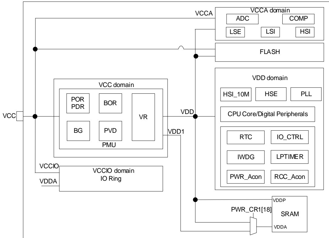
图 2-2 电源框图
