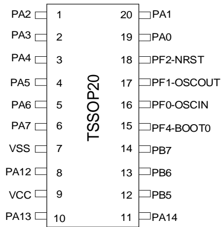
图 3-13 TSSOP20 Pinout2 PY32F030F2xP
