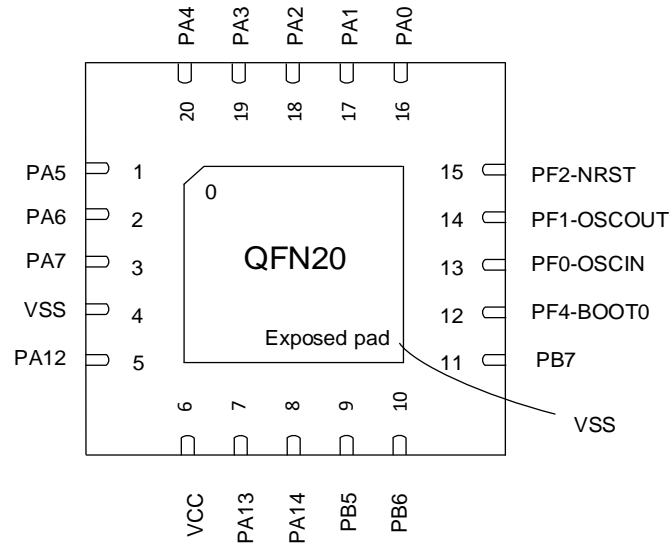
图 3-10 QFN20 Pinout2 PY32F030F2xU / PY32F030F2xU -E
