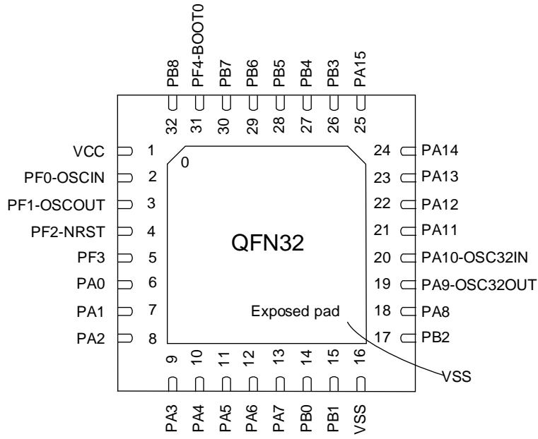
图 3-3 QFN32(5*5) Pinout2 PY32F030K2xU / PY32F030K2xU -E
