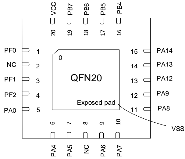
图 3-11 QFN20 Pinout3 PY32F030F3xU
