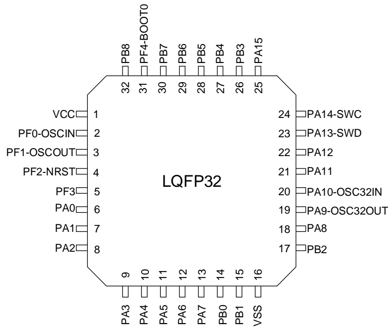
图 3-2 LQFP32 Pinout2 PY32F030K2xT / PY32F030K2xT-E
