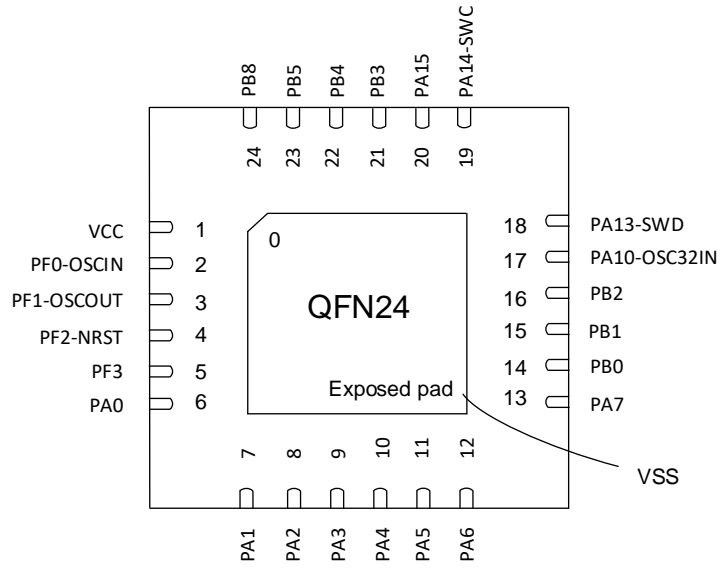
图 3-8 QFN24 Pinout1 PY32F030E1xU-E
