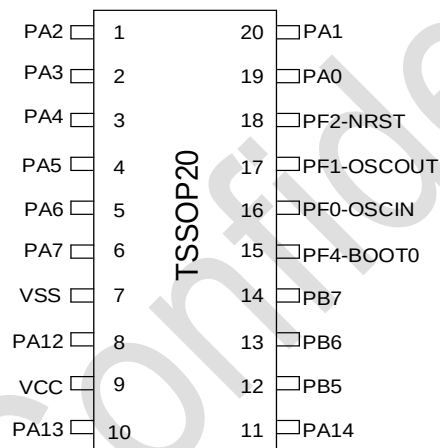
图 3-13 TSSOP20 Pinout2 PY32F030F2xPx (Top view)
