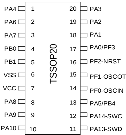
图 3-15 TSSOP20 Pinout4 PY32F030F4xPx (Top view)
