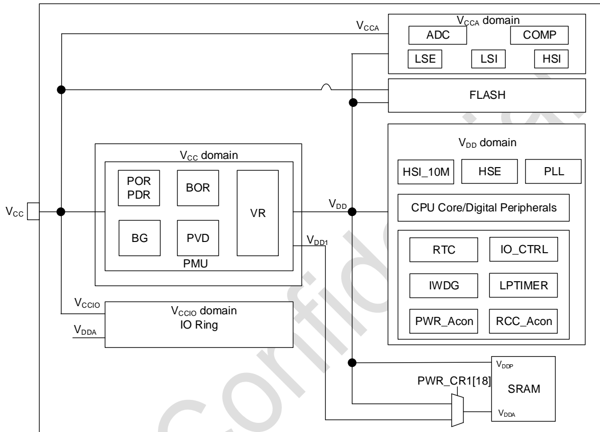
图 2-2 电源框图
