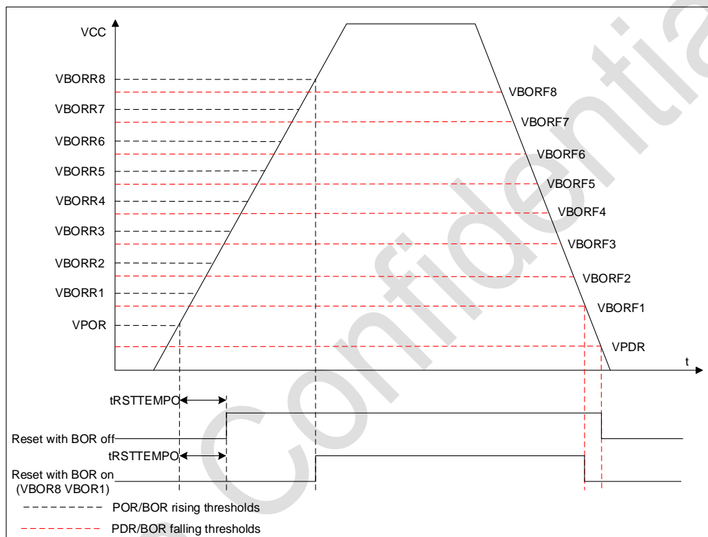
图 2-3 POR/PDR/BOR 阈值
